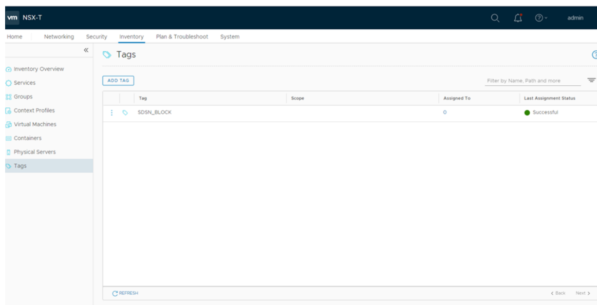
Figure 85: Tags Page
