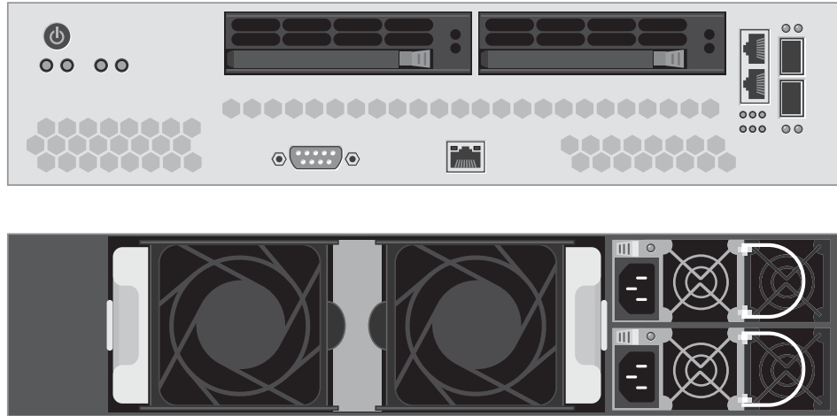
圖 1: Secure Access 6000 前面板與後面板
